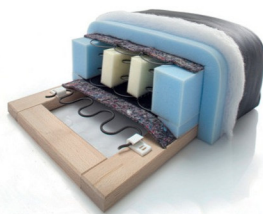
Federkern-Aufbau
